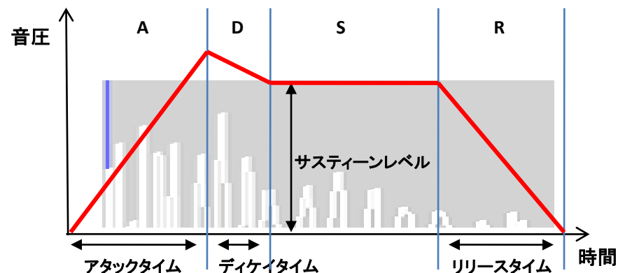
ADSR方式のエンベローブ
